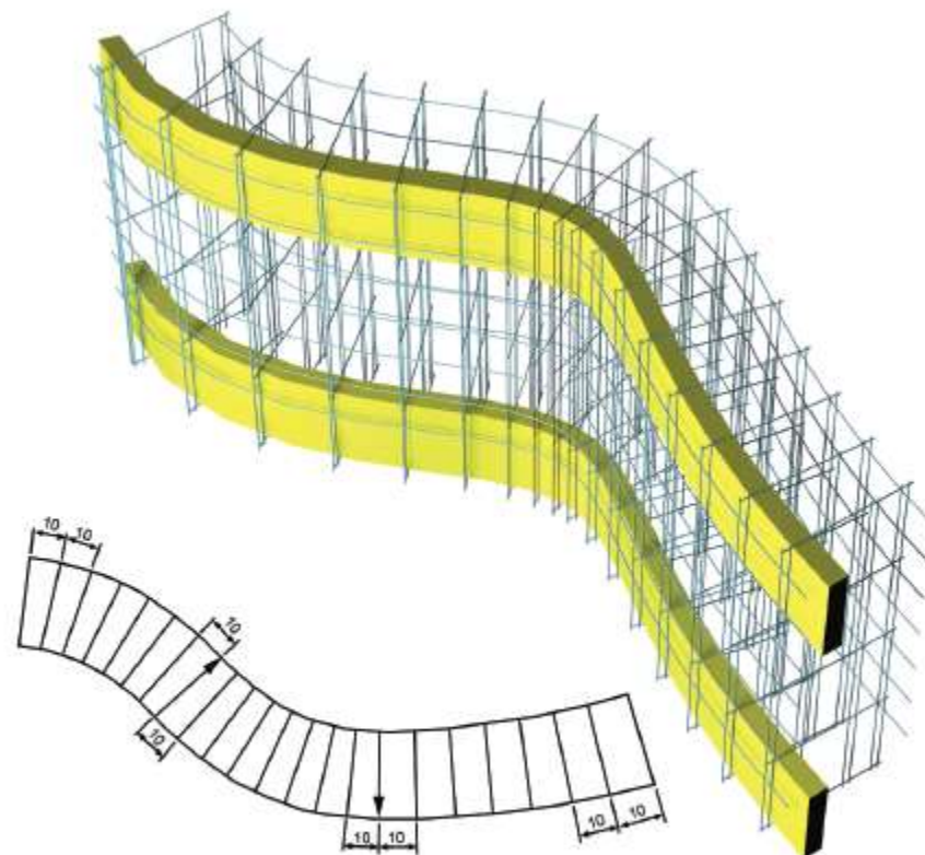
Il modulo ECOSISM può essere curvato.
