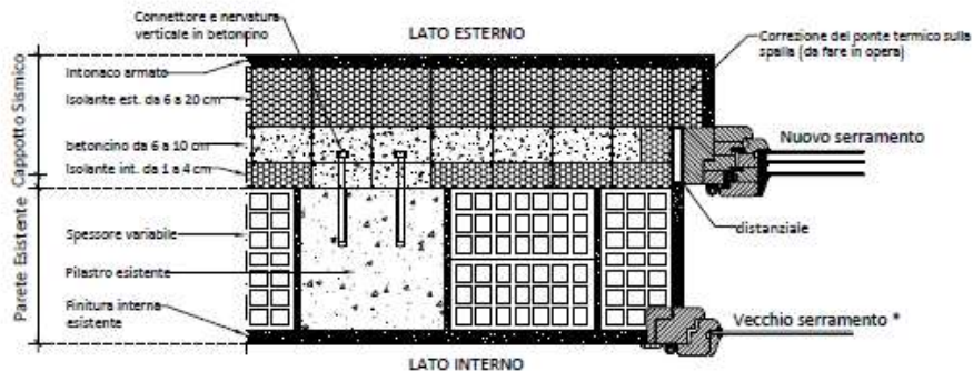
Esempio 2 - Con sostituzione del vecchio serramento
