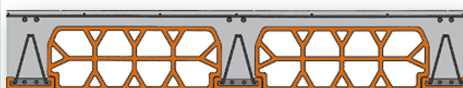
Solaio latero-cemento - 20+4
