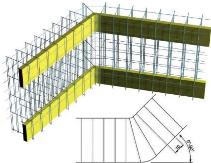
Il modulo ECOSISM può essere piegato.
