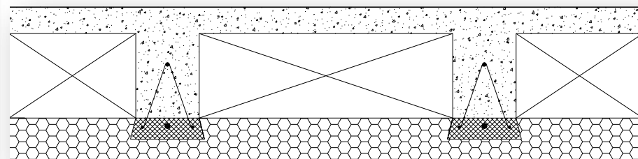
ECOSOLAIO TOP - 4+4+16+4 (20+4)
