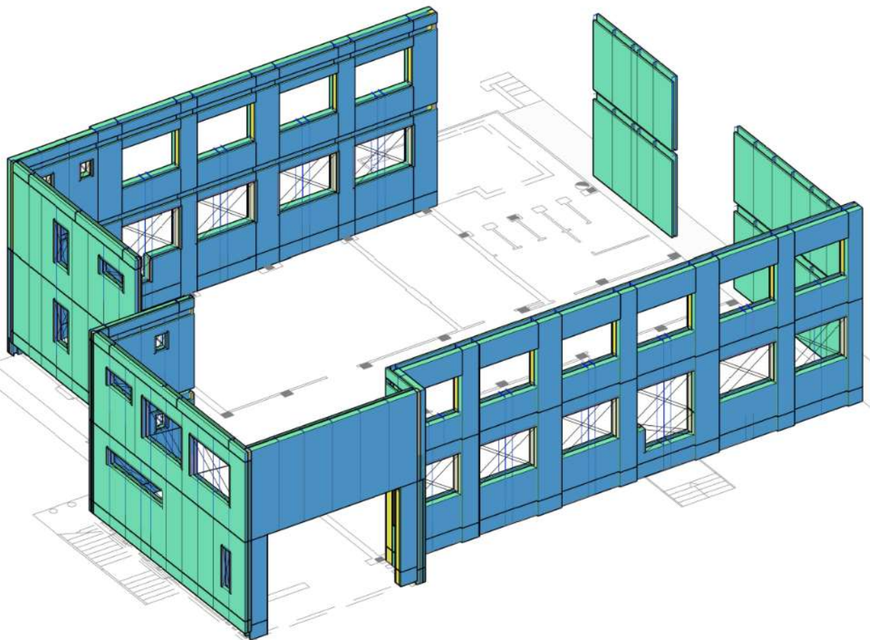
Modello 3D di produzione Ecosism
