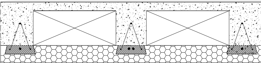
ECOSOLAIO - 4+4+16+4 (20+4)
