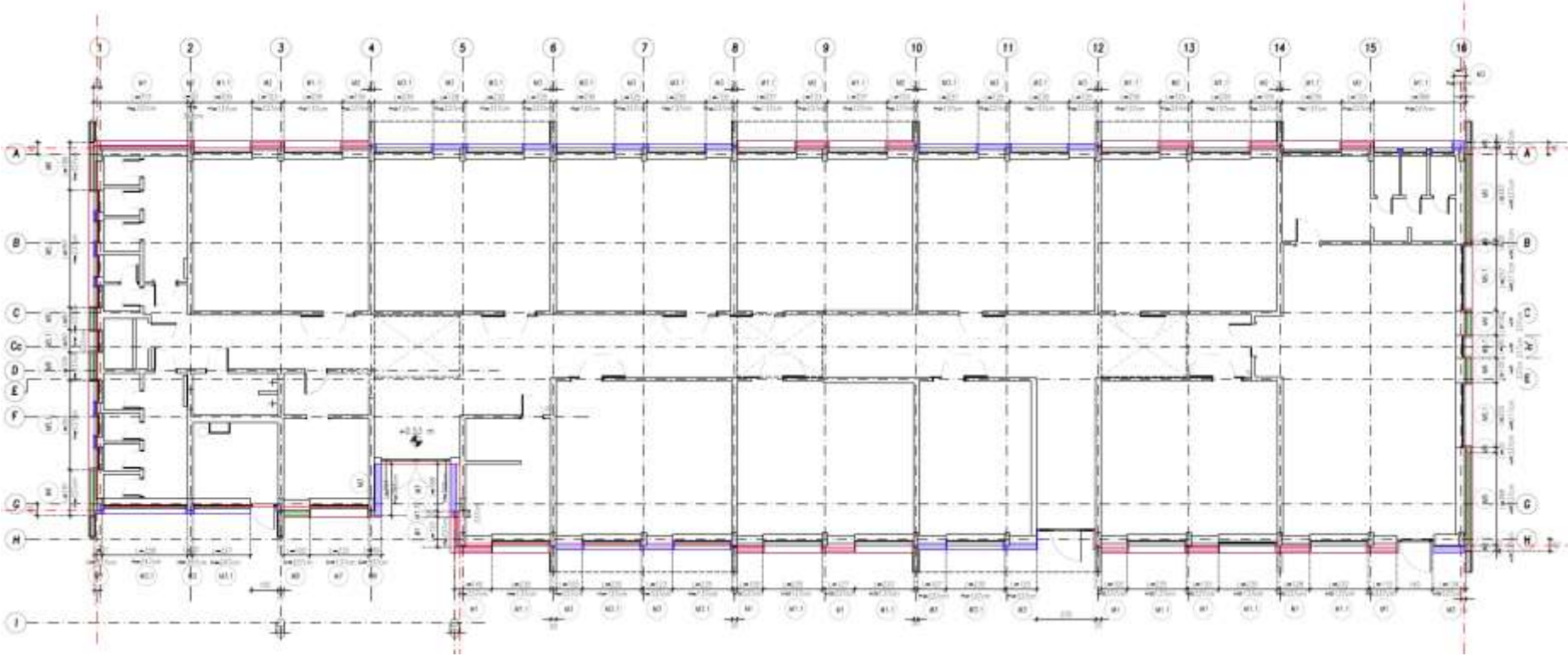
PIANTA CHIAVE 1 - STRATIGRAFIA NUOVE PARETI da quota +0.00 a +3.37 m SCALA 1:100
