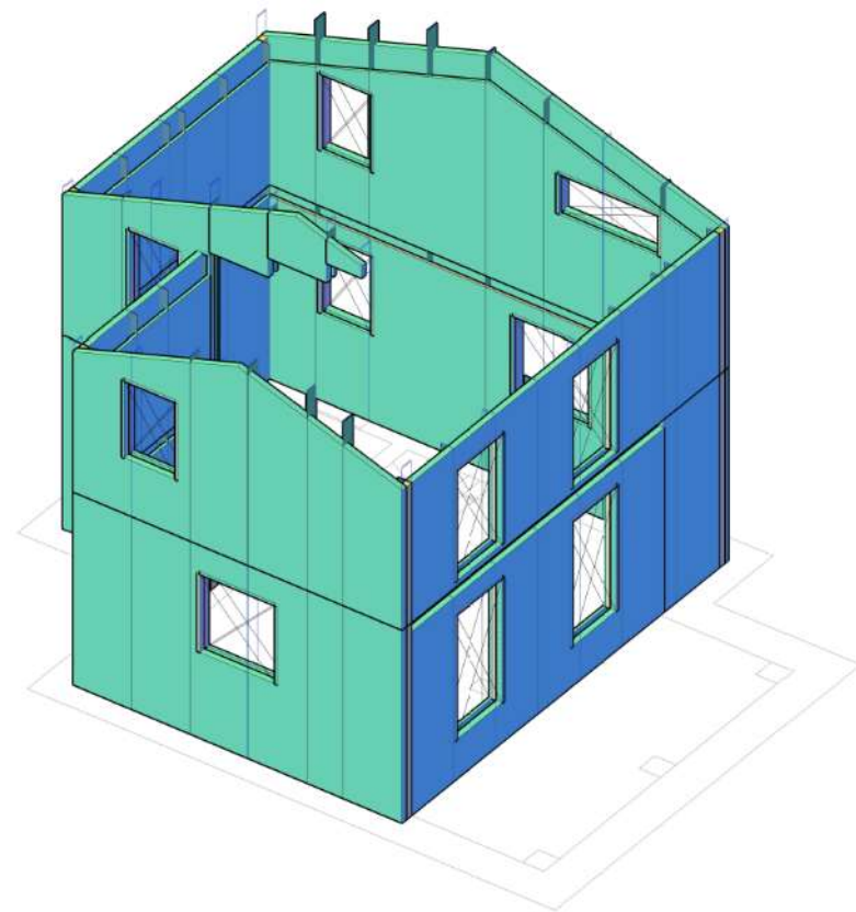
Modello 3D di produzione Ecosism
