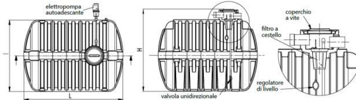
Filtro a cestello
