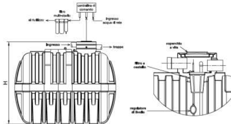
Filtro a cestello
