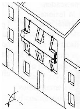
Fig. 1.2 – Meccanismi di flessione verticale (Foto da: MEDEA - Zuccaro, Papa - 2003, DPC)
